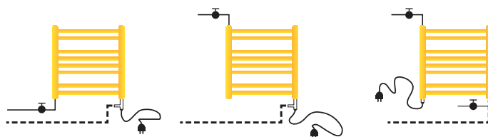
Примеры схем подключения электрического нагревательного элемента GRZ к радиатору
